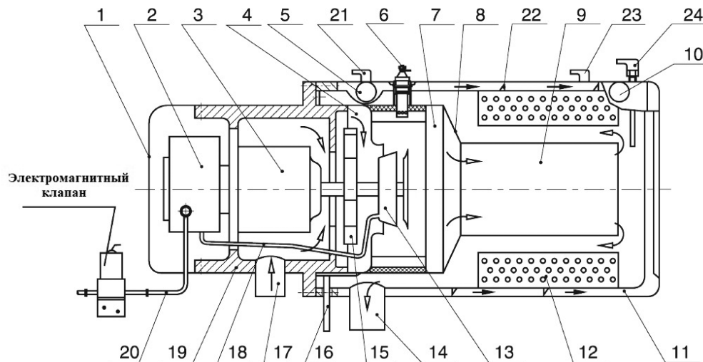
Рис.2. Устройство предпускового жидкостного догревателя YJ-Q35
