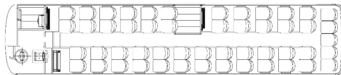
Расположение сидений для 52TR1 (51+1+1) с диспенсером для воды
