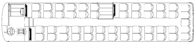
Расположение сидений для 52TR1 (51+1+1)
