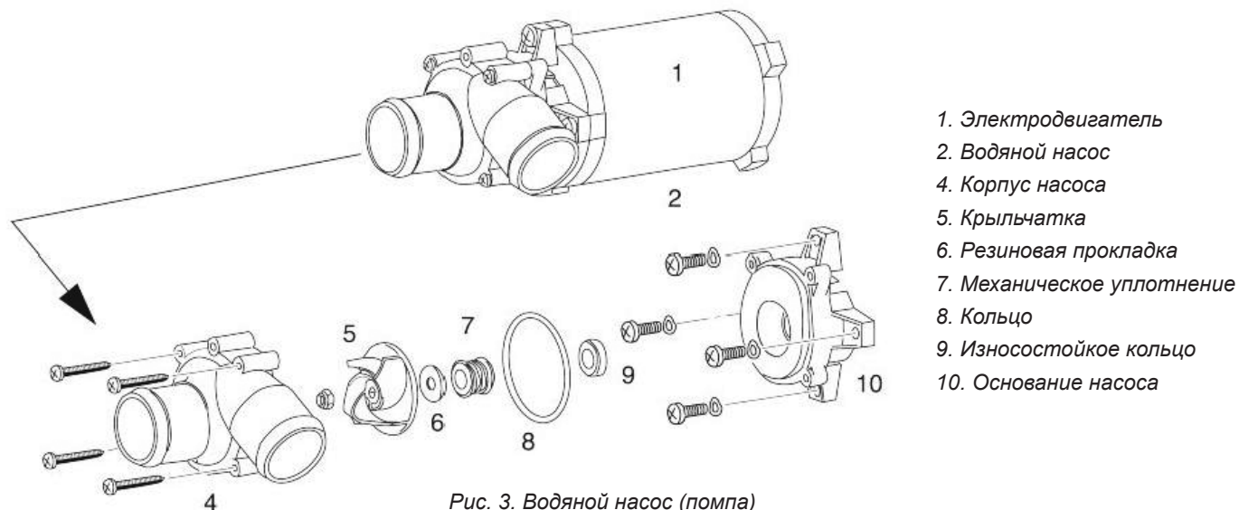
Рис. 3. Водяной насос (помпа)
