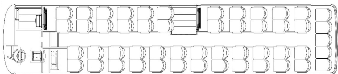
Расположение сидений для 52TR1 (51+1+1) с холодильником
