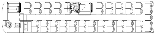
Расположение сидений для 52TR2 (49+1+1) с холодильником и туалетом
